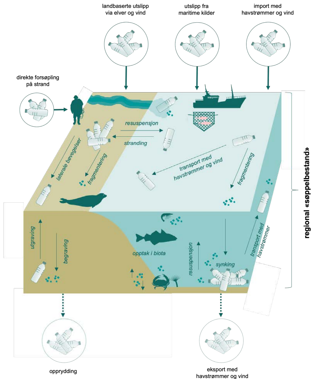
Figur 77: Skjematisk fremstilling av et «søppelbudsjett» med prosesser som tilfører søppel, omdistribuerer søppel i systemet, og prosesser som fjerner søppel fra regionen. Dette representerer variabler som må estimeres for å parametrisere en massebalansemodell.
